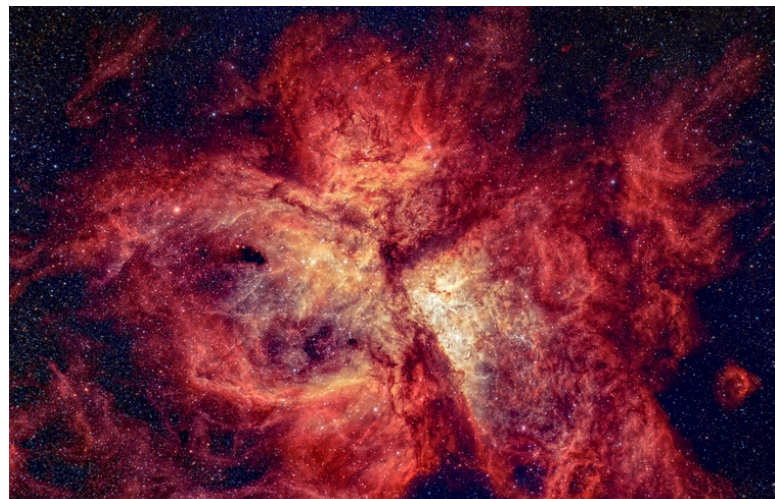
eta carina nebula
